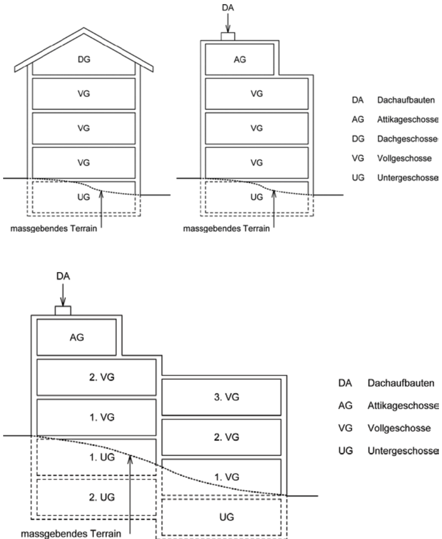
Figur 5.1 Geschosse und Geschosshzahl
