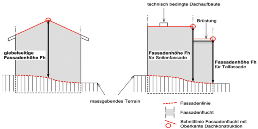
Figur 4.2.b Fassadenhöhe
