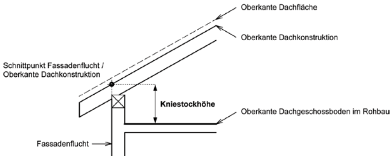
Figur 4.3 Kniestockhöhe
