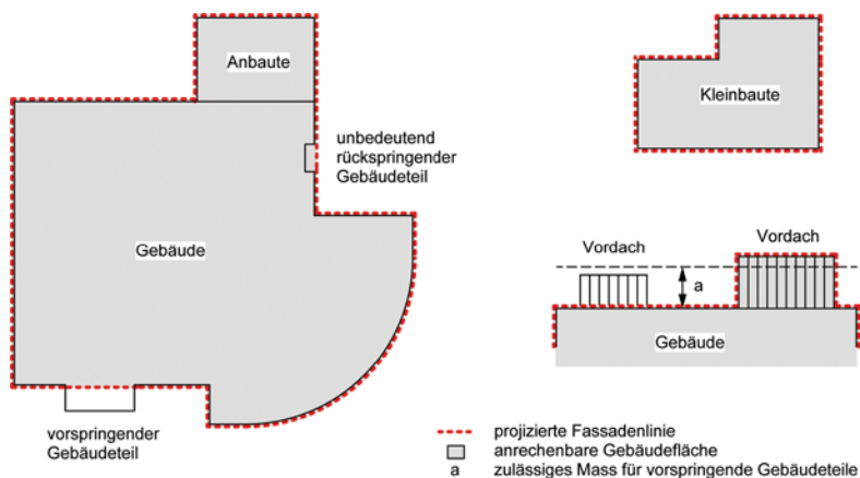
Figur 7.4 Anrechenbare Gebäudefläche
