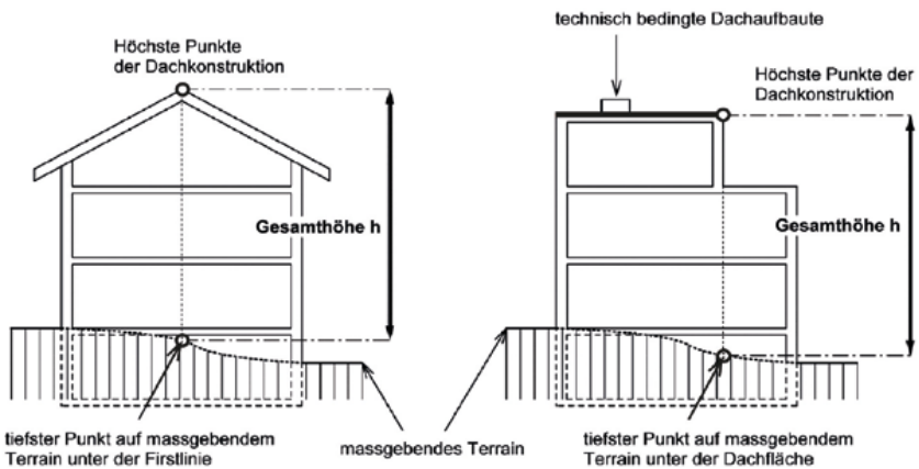
Figur 4.1.a Gesamthöhe
