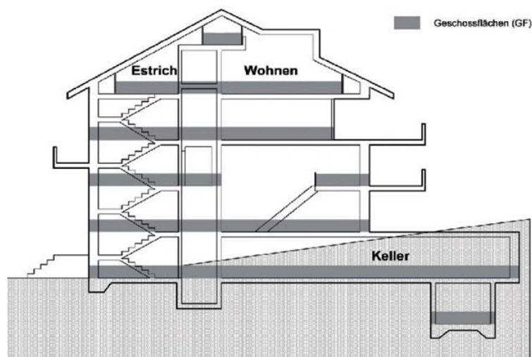
Figur 7.2 Geschossflächenziffer
