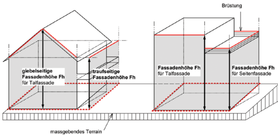
Figur 4.2.a Fassadenhöhe
