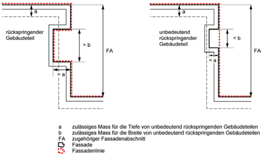
Figur 2.4 Rückspringende und unbedeutend rückspringende Gebäudeteile
